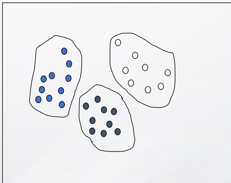
Raw Data
