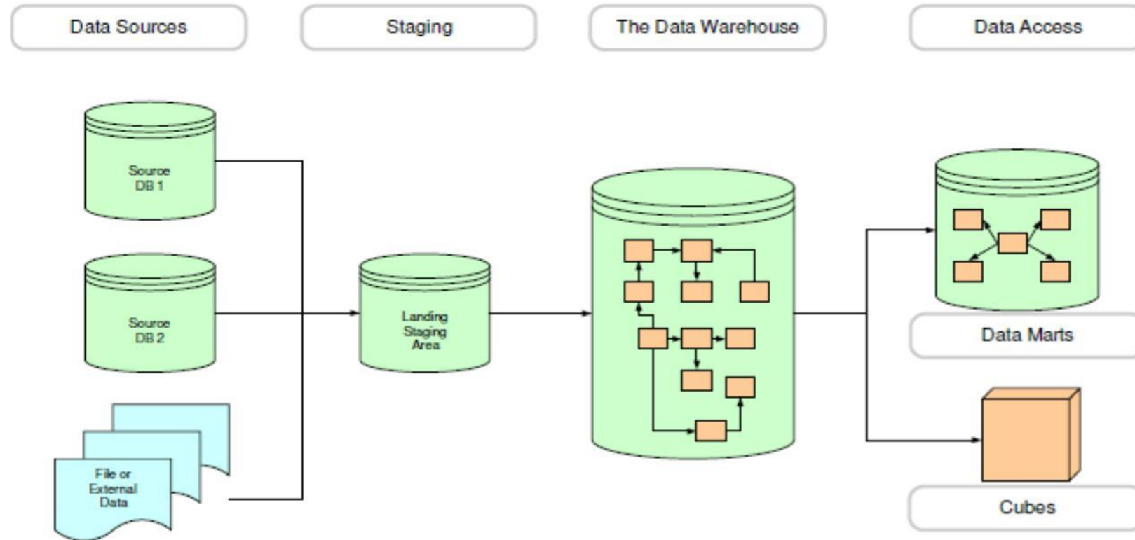
Inmon Model
