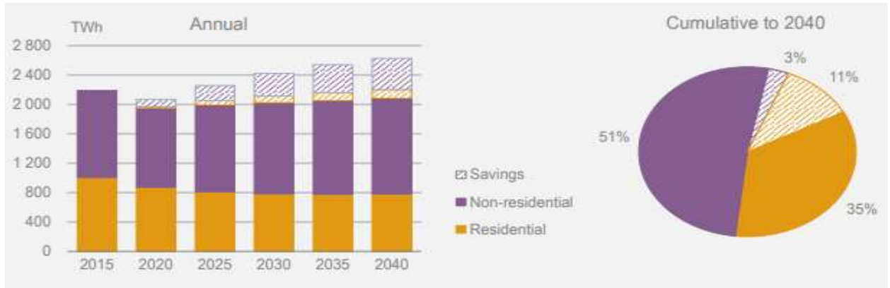
الشكل 7 التوفير المتوقع للطاقة عند استخدام نظام الإنارة الذكي في 2040 (المصدر: (IEA, 2017))
