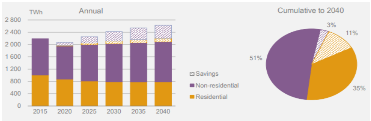
الشكل 8 التوفير المتوقع للطاقة عند استخدام نظام الإنارة الذكي في 2040 (المصدر: (IEA, 2017))
