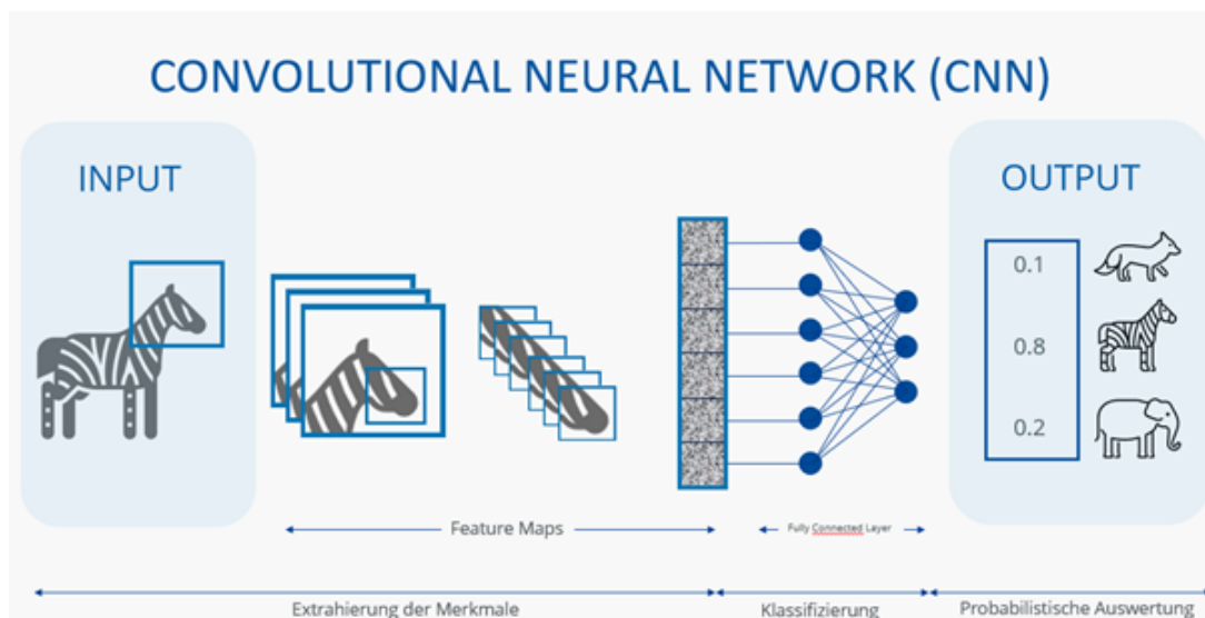
Fig. 3. CNNs
