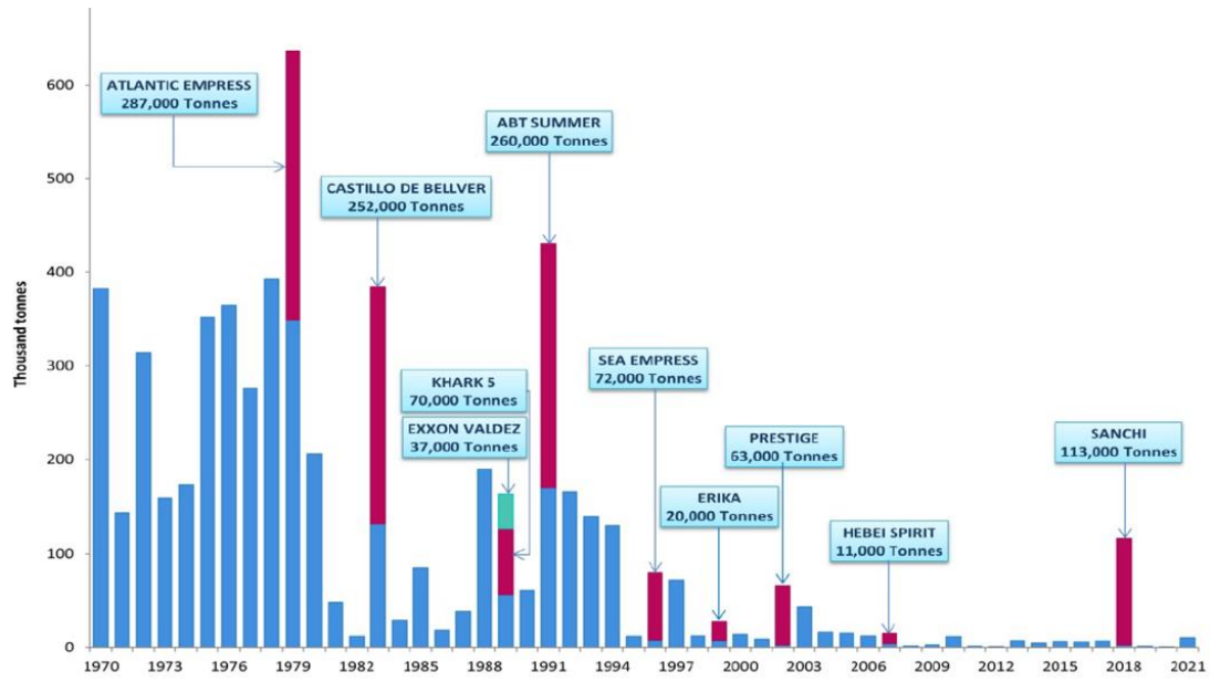
الشكل رقم (١٠): يمثل كمية الانسكاب النفطية مع توضيح أسماء الناقلات.
