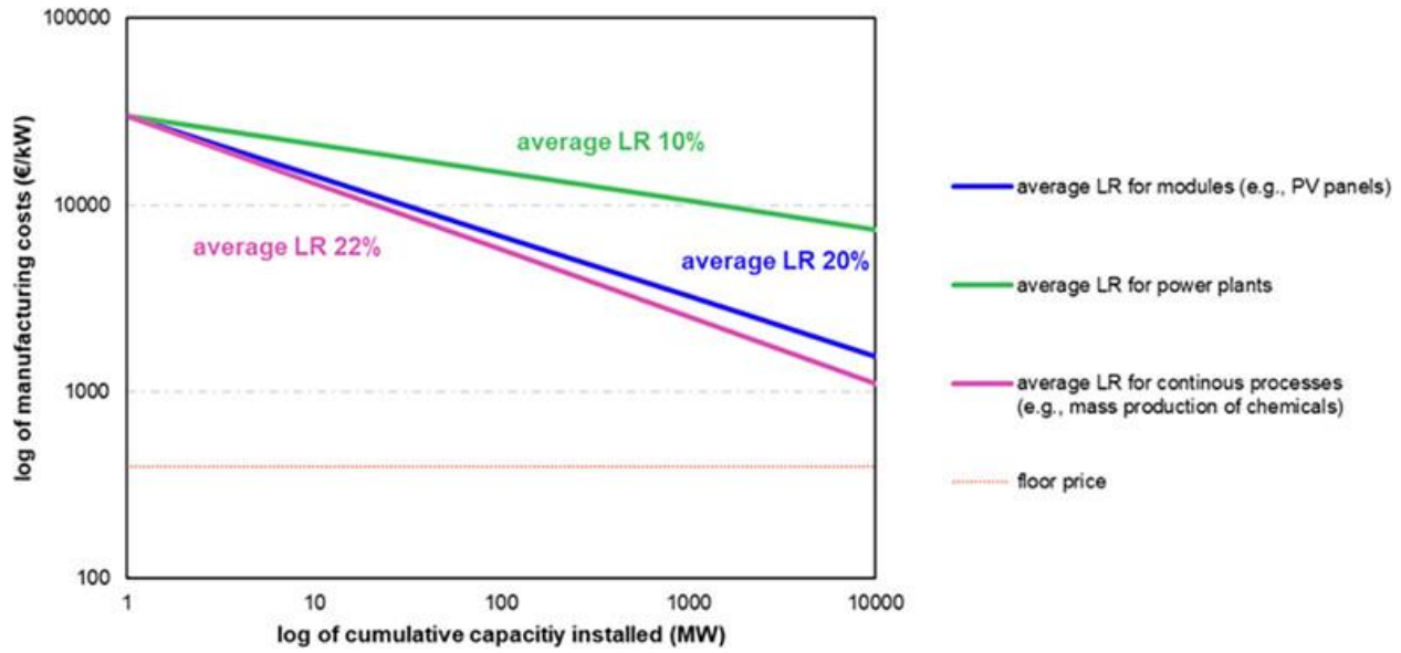
الشكل 4 منحنى الخبرة/ التعلم لتكاليف مشاريع الطاقة الشمسية (المصدر (Hass et al., 2023))
