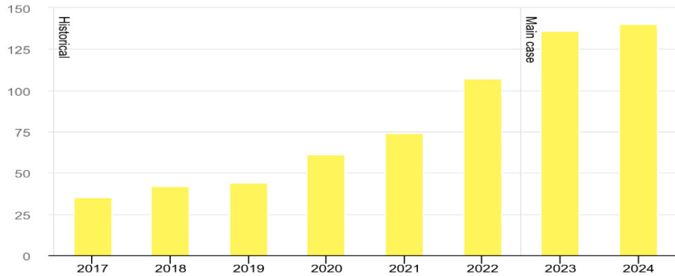
الشكل 3 تزايد استخدام الطاقة الشمسية من 2017-2024 (المصدر: (IEA, 2023))
