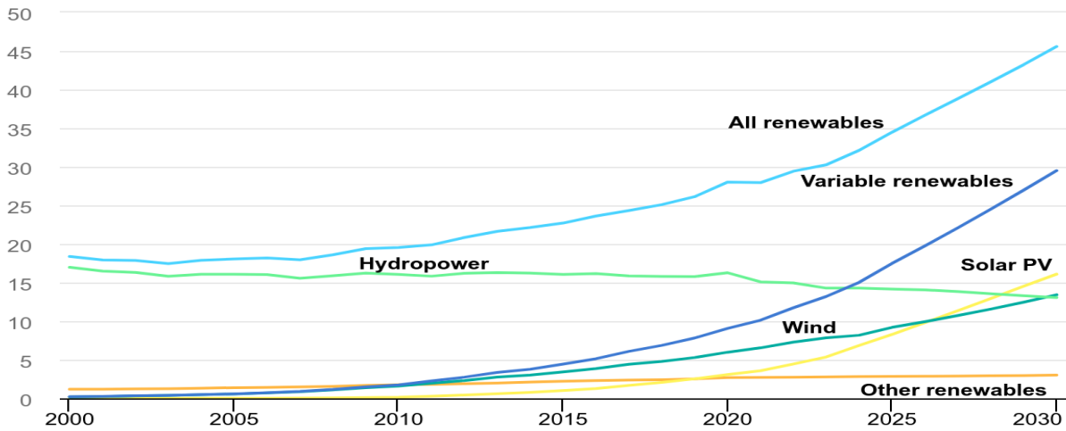
الشكل 6 مخطط إنتاج الطاقة المتجددة حسب التقنية من 2000-2030 (المصدر: (IEA, 2023))
