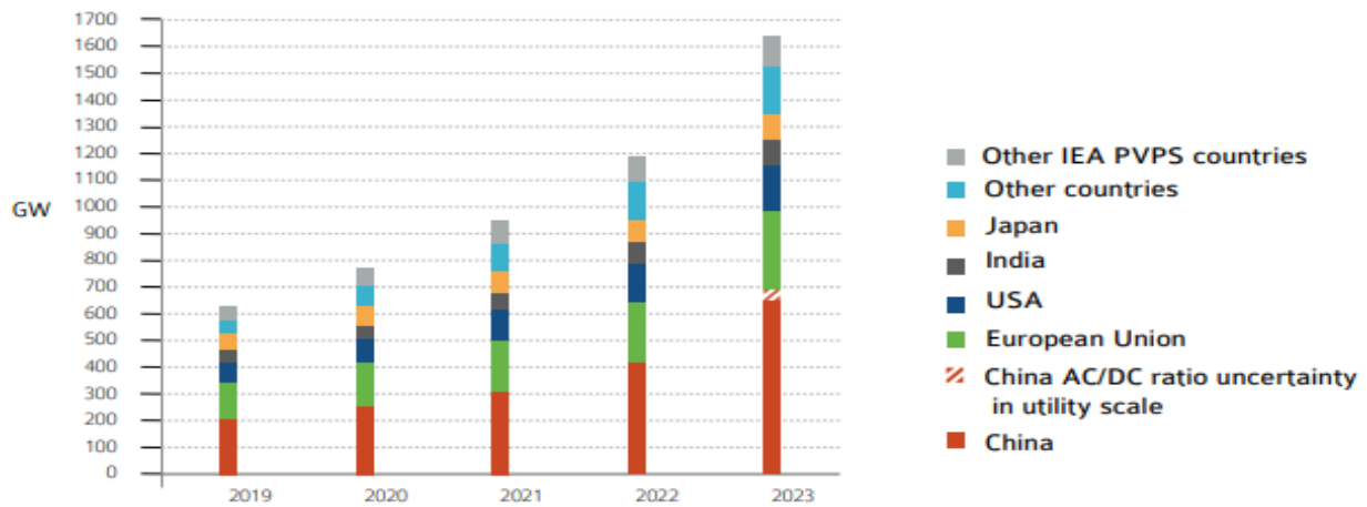
الشكل 5 نمو استخدام الطاقة الشمسية في الأسواق من 2018-2023 (المصدر: (IEA, 2023))
