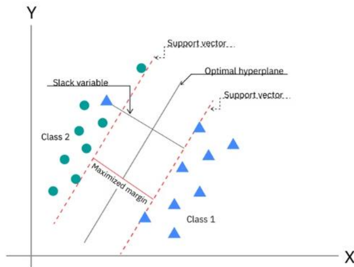
Fig.6. SVM [27].
