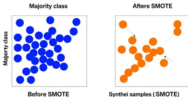
Fig. 15 SMOTE
