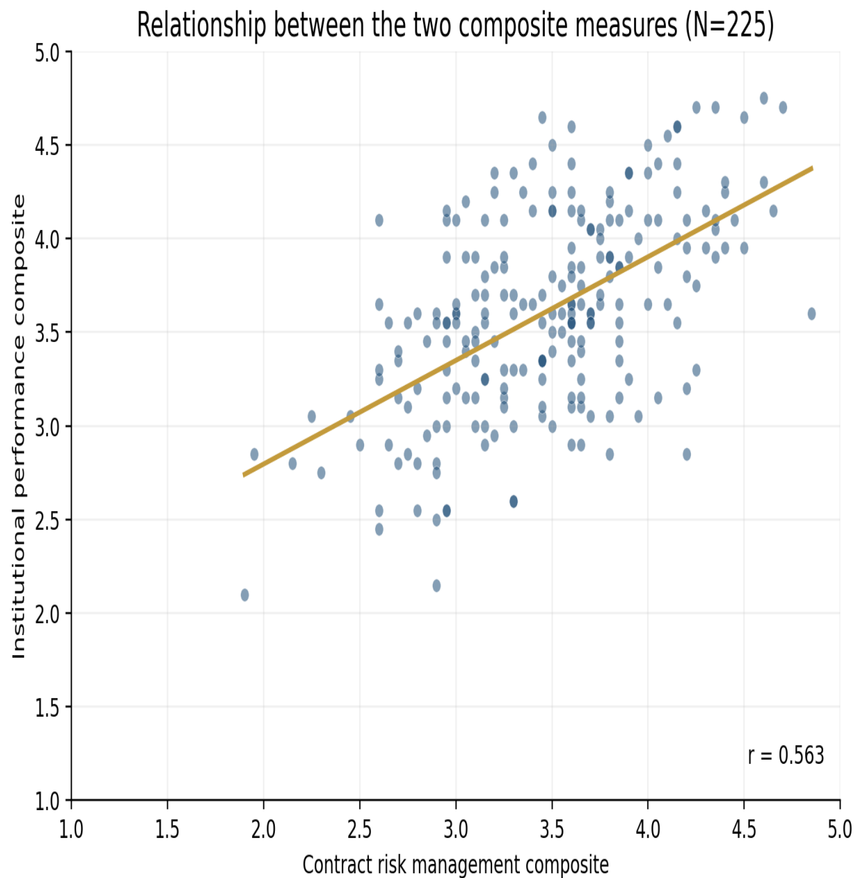
شكل 3 العلاقة بين المتوسطين المركبين — كل نقطة تمثل استجابة واحدة؛ المصدر: تحليل بيانات الدراسة
