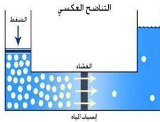
شكل ١ اليه فلتر المياه باستخدام تقنية التناضح العكسي
