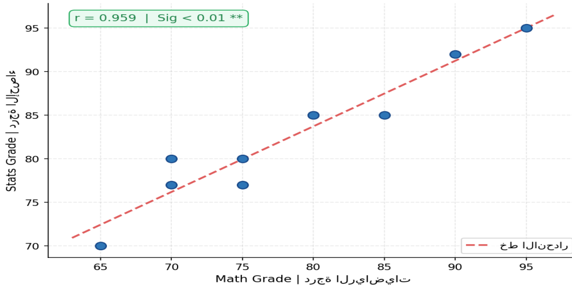
Scatter Plot: Math vs Stats | r = 0.959 (أصاح إل أو تايضاي رلا: راش تنال ططخ م)
