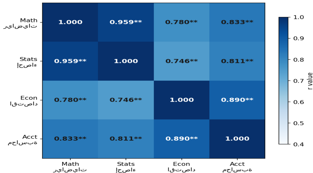
Correlation Matrix | طابترالالاماعم ةفوفصم (نمائلال فيلكللال ةلعلالالانايال)
