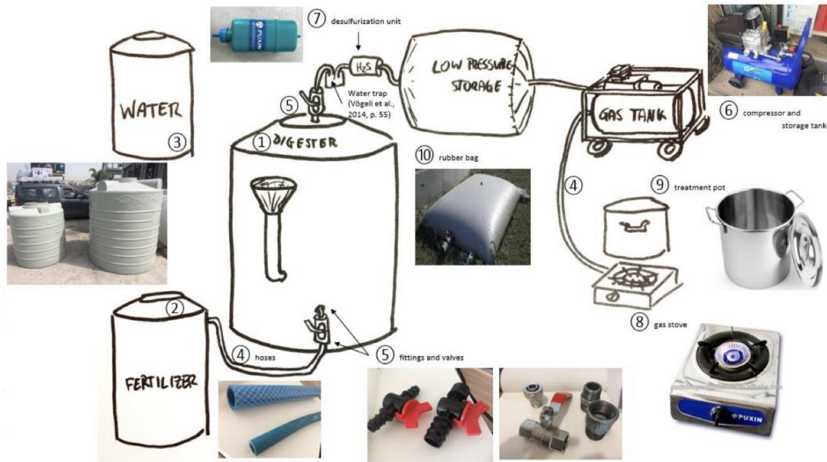
Huber et al 2019 شكل ١١: مكونات تجميع مفاعل الغاز الحيوي في الدراسة -
